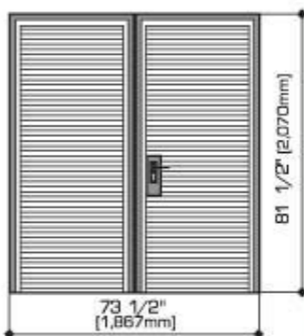
Fixed Louvred Double Door
